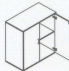
NY-8822/W Swinging Door Cabinet L800 x W400 x H835 mm
